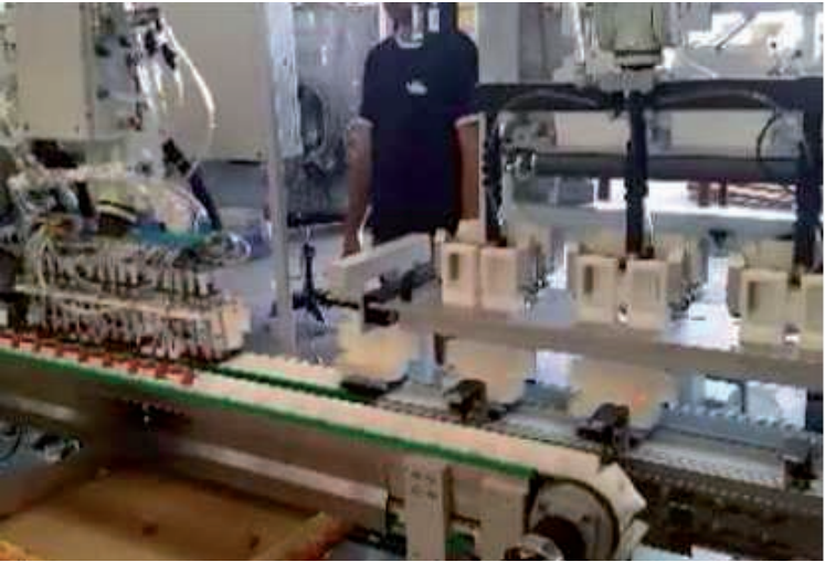
Etuis à partir de découpe à plat Cadence mise en étuis 40/min
