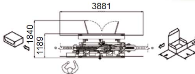
Plan fermeuse type pour box 1 seul rabat (BC1) (version miroir disponible)
