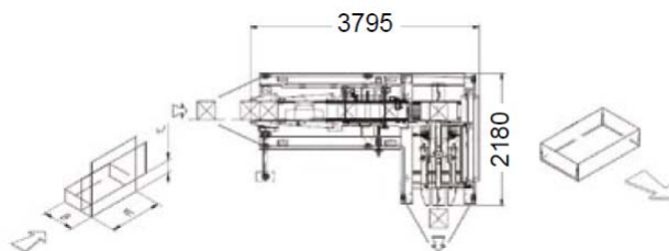
Plan fermeuse type pour box 3 seul rabats (BC3) (version miroir disponible)
