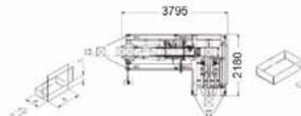
Plan fermeuse type pour box 3 seul rabats (BC3) (version miroir disponible)
