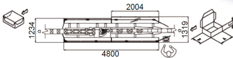
Plan fermeuse type pour box 3 rabats (BC3) (version miroir disponible)
