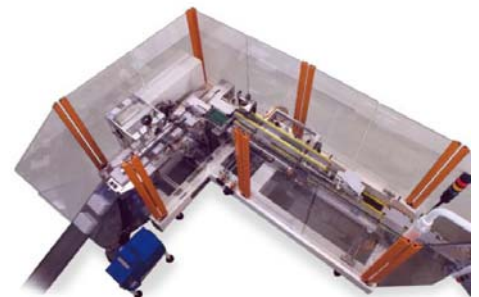
Plan fermeuse type pour box 3 seul rabats (BC3) (version miroir disponible)
