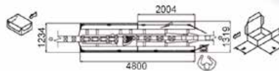
Plan fermeuse type pour box 3 rabats (BC3) (version miroir disponible)
